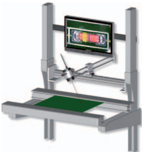
Configuration B : Caméra HD sur ligne avec moniteur Full HD 22", supports flottants XY et module d'inclinaison dans 4 directions.
